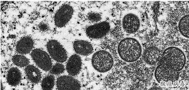
猴痘病毒
